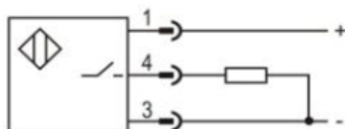
PNP NO
