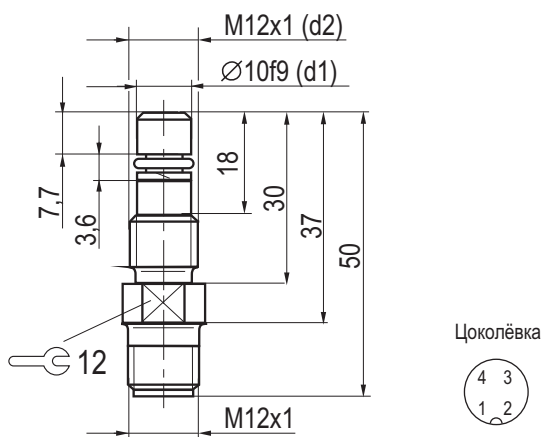
Схема монтажа
