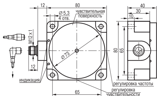
Габаритный чертеж
