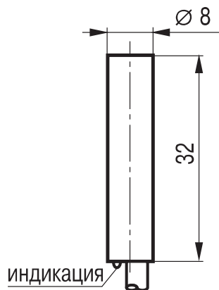
Габаритный чертеж
