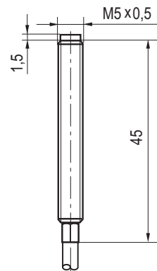
Габаритный чертеж
