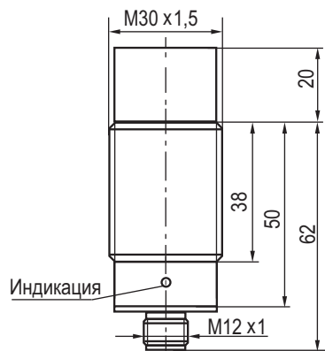
Габаритный чертеж
