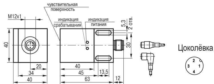
Габаритный чертеж
