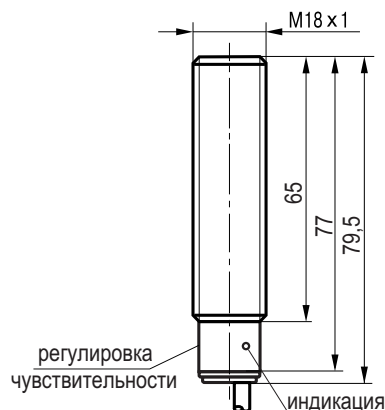
Габаритный чертеж.
