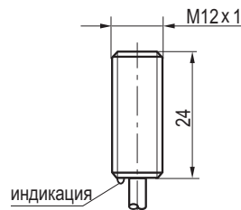
Габаритный чертеж
