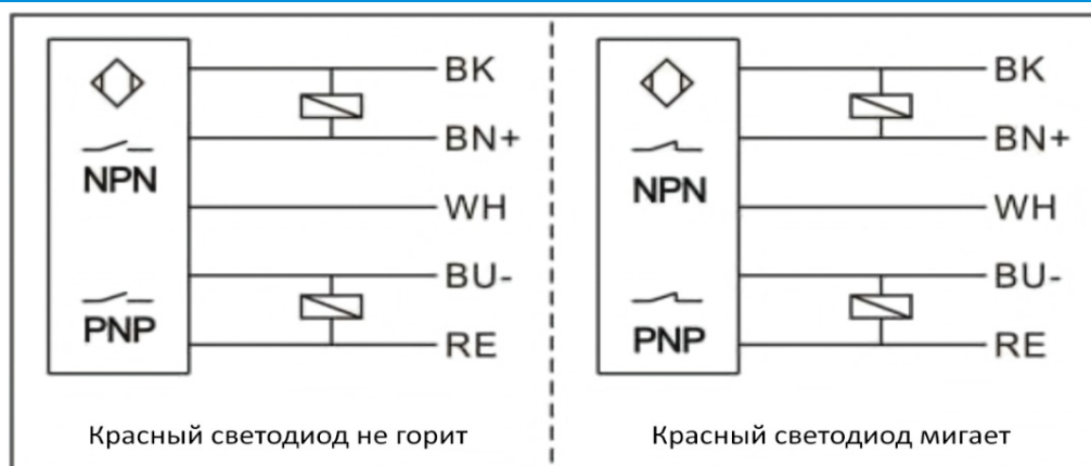
Схема подключения
