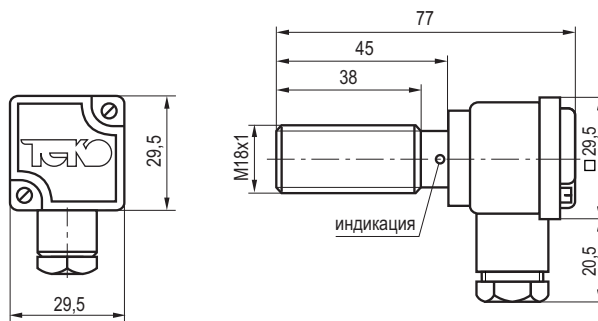
Габаритный чертеж
