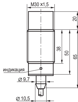
Габаритный чертеж
