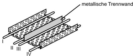
Alternativ: Leitungen durch metallischen Trennsteg trennen
