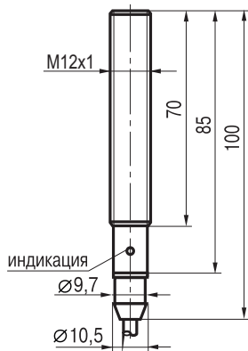
Габаритный чертеж
