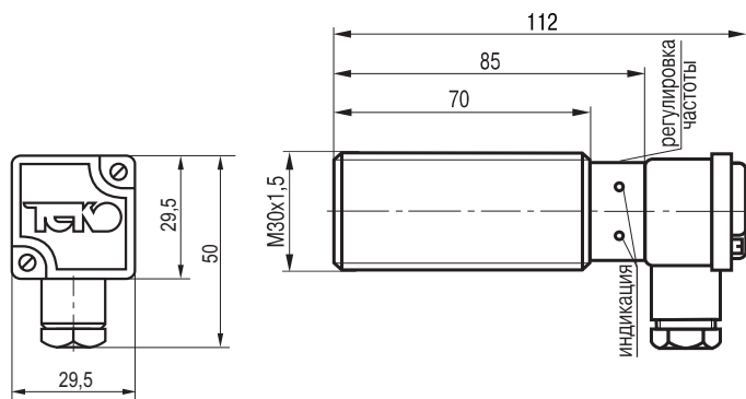
Габаритный чертеж
