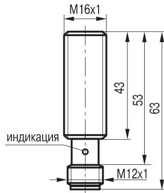
Габаритный чертеж
