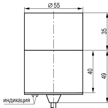
Габаритный чертеж
