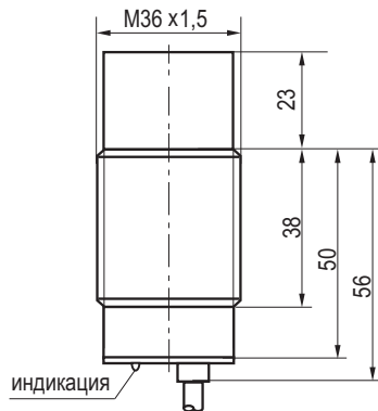
Габаритный чертеж
