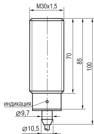
Габаритный чертеж
