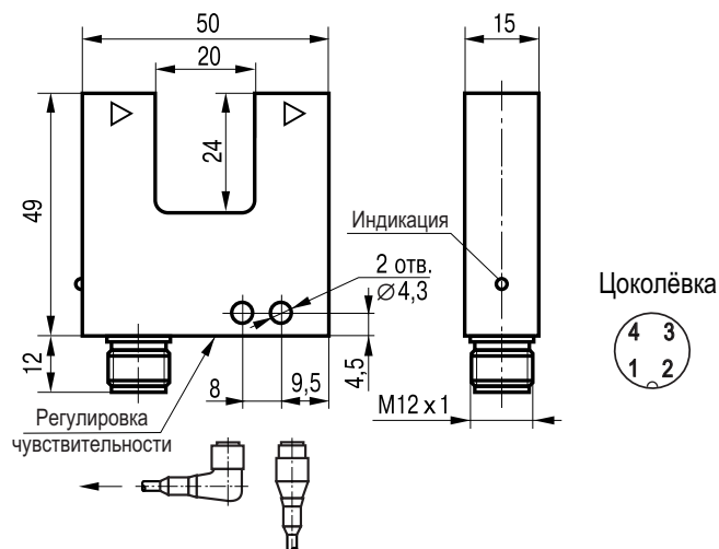
Габаритный чертеж
