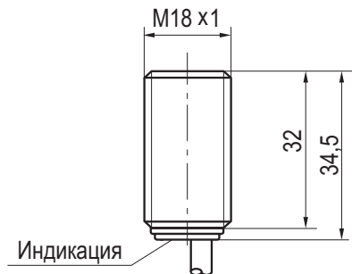
Габаритный чертеж
