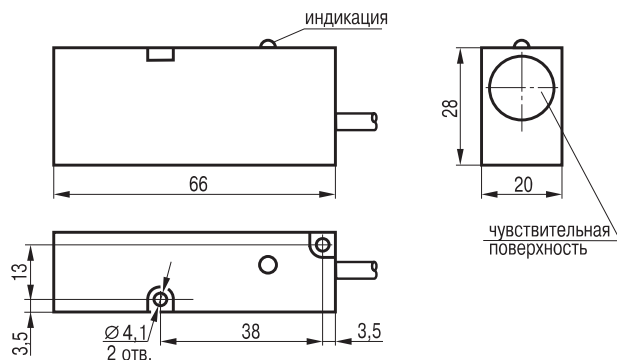
Габаритный чертеж
