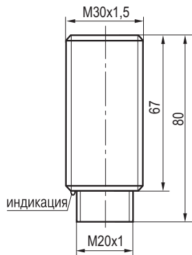
Габаритный чертеж
