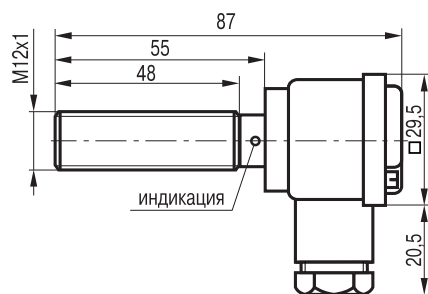
Габаритный чертеж
