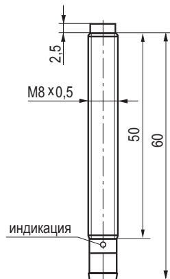
Габаритный чертеж
