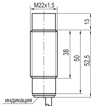
Габаритный чертеж
