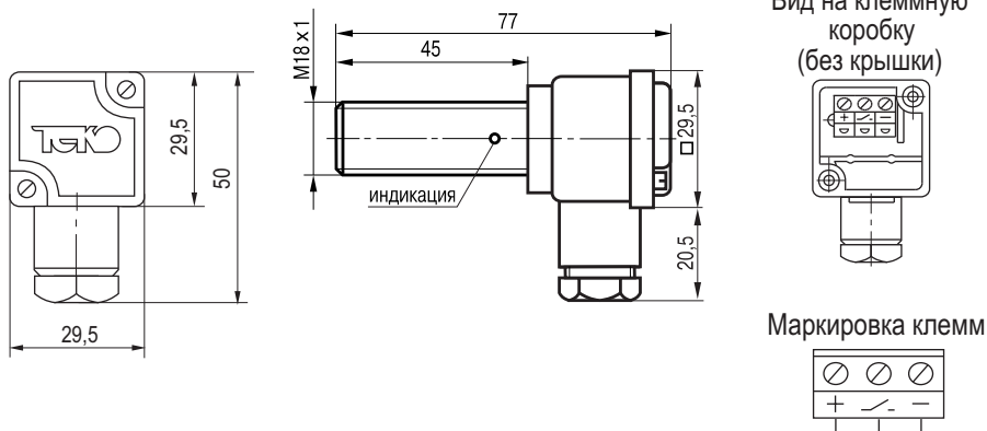
Габаритный чертеж.
