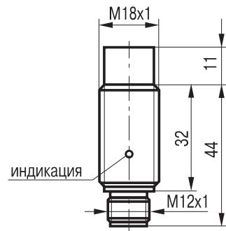
Габаритный чертеж
