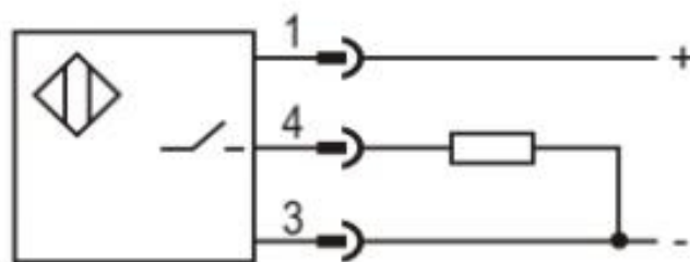
PNP NO
