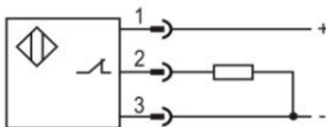
PNP NO
