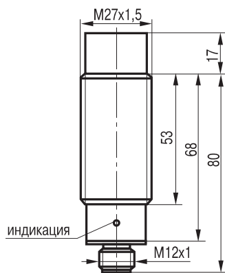
Габаритный чертеж
