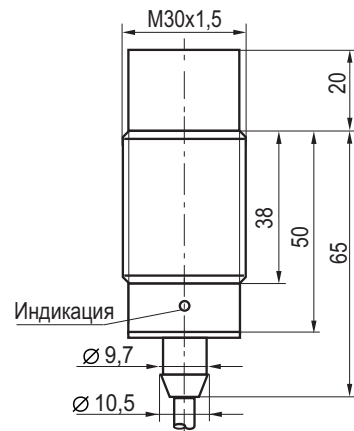
Габаритный чертеж
