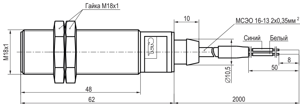
Габаритный чертеж
