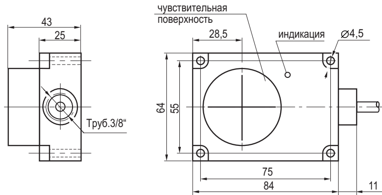
Габаритный чертеж
