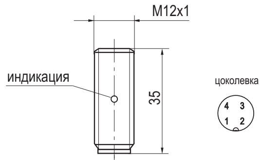
Габаритный чертеж
