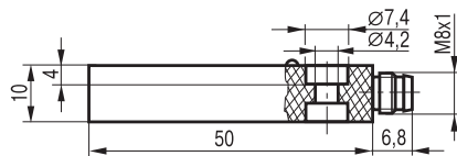
Габаритный чертеж
