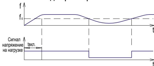
Диаграмма работы
