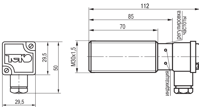
Габаритный чертеж
