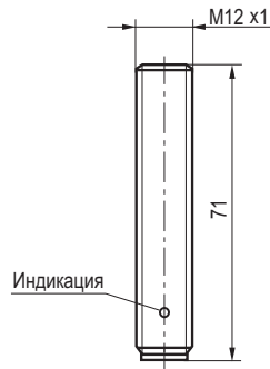
Габаритный чертеж
