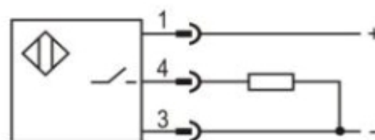
PNP NO
