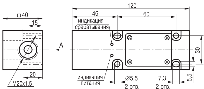
Габаритный чертеж
