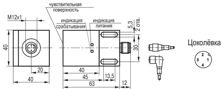
Габаритный чертеж
