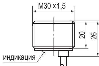
Габаритный чертеж
