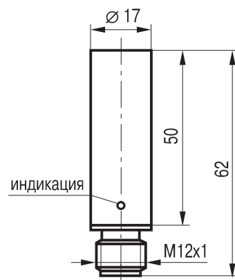
Габаритный чертеж
