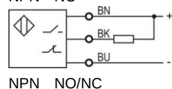
NPN NO/NC
