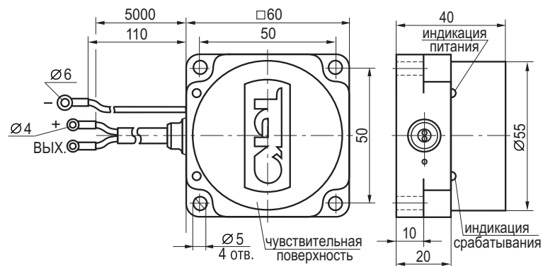
Габаритный чертеж
