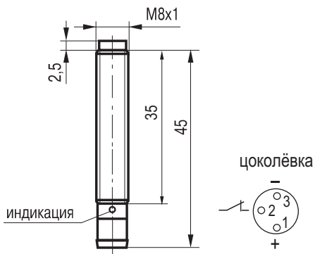
Габаритный чертеж
