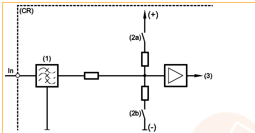
Grafik: Prinzipschaltung Binäreingang minus-schaltend / plus-schaltend für negative und positive Gebersignale
