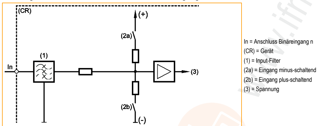
Grafik: Prinzipschialtung Binäreingang minus-schaltend / plus-schaltend für negative und positive Gebersignale
