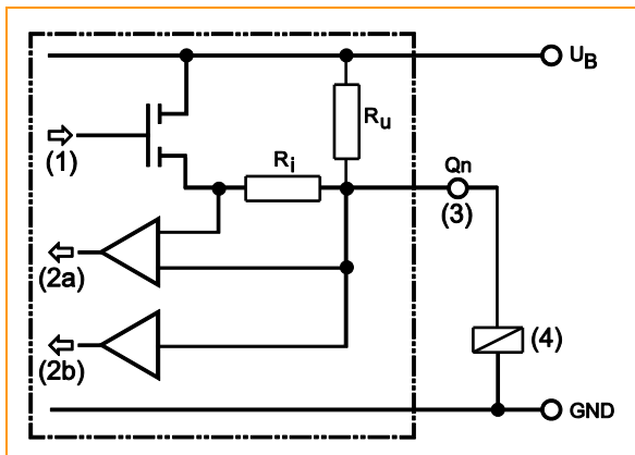
Grafik: Prinzipschaltung
