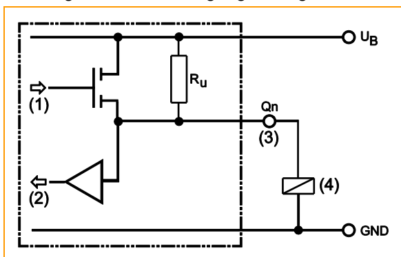
Grafik: Prinzipschaltung
