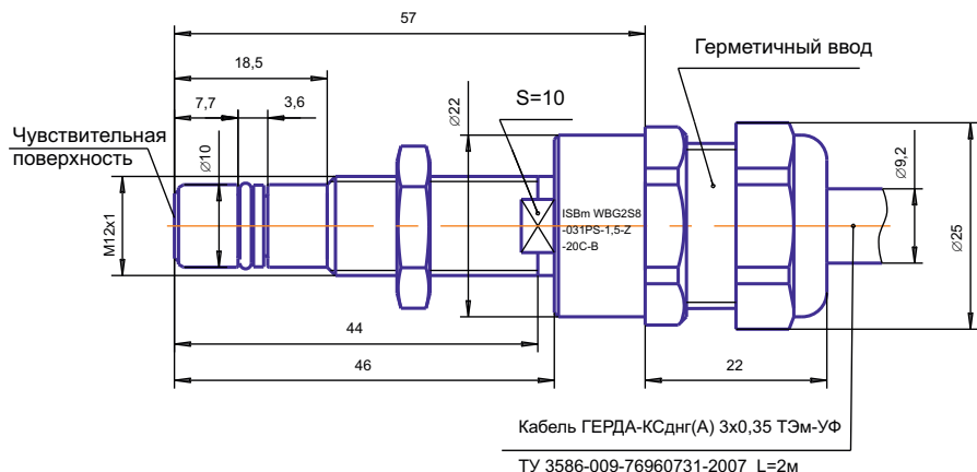
Габаритный чертеж
