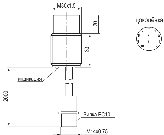
Габаритный чертеж
