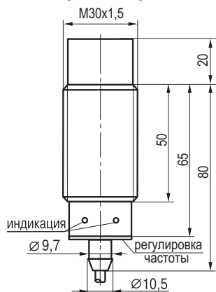
Габаритный чертёж
