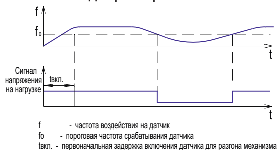
Диаграмма работы
