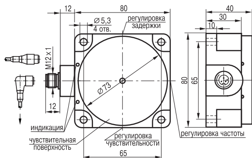
Габаритный чертеж
